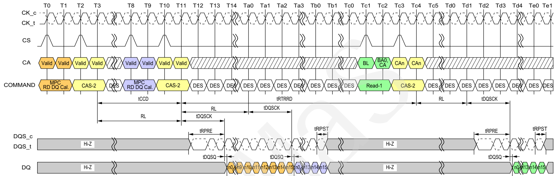
Figure 110 - DQ Read Training Timing: Read DQ Cal. to Read DQ Cal. / Read
