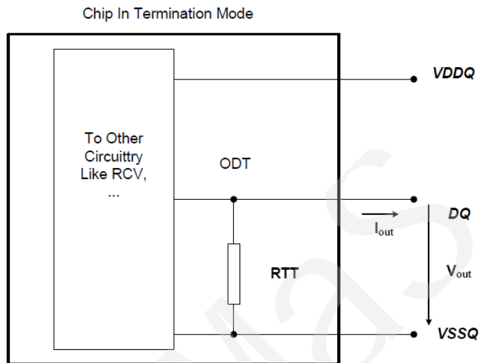
Figure 133 - DQ On Die Termination
